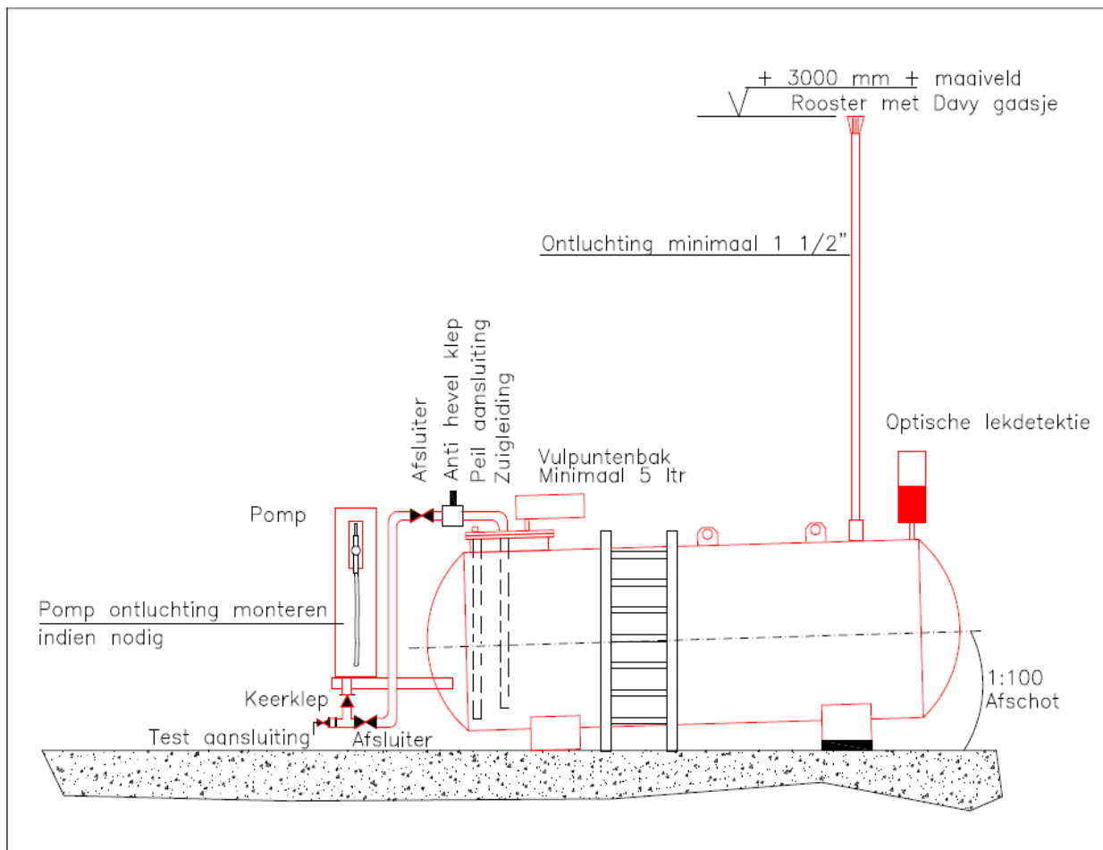
Figuur 13.1: Voorbeeld van antihevelvoorziening in bovengrondse tankinstallatie
